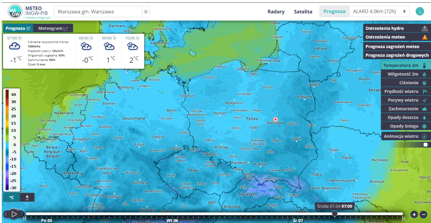
Temperatura powietrza w środę 07.04.2021 w Europie.
