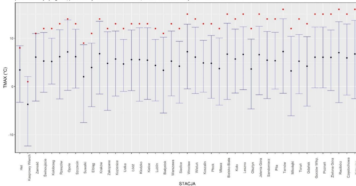
Prognoza wartości TMAX (2024-03-01) na tle warunków wieloletnich (1991-2020). Kolejność stacji według różnicy TMAX prognoza – TMAX z wielolecia.
