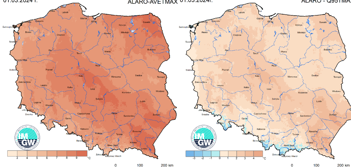
Anomalia prognozy TMAX (2024-03-01) względem notowanych charakterystyk wieloletnich (1991-2020): ALARO-AVETMAX – ALARO-wartość średnia TMAX (po lewej), ALARO-Q95TMAX – ALARO-kwantyl 95% TMAX (po prawej).
